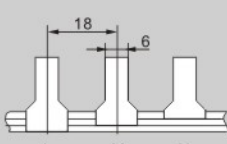
DZ47-3P
