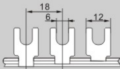
LFL7-3P
